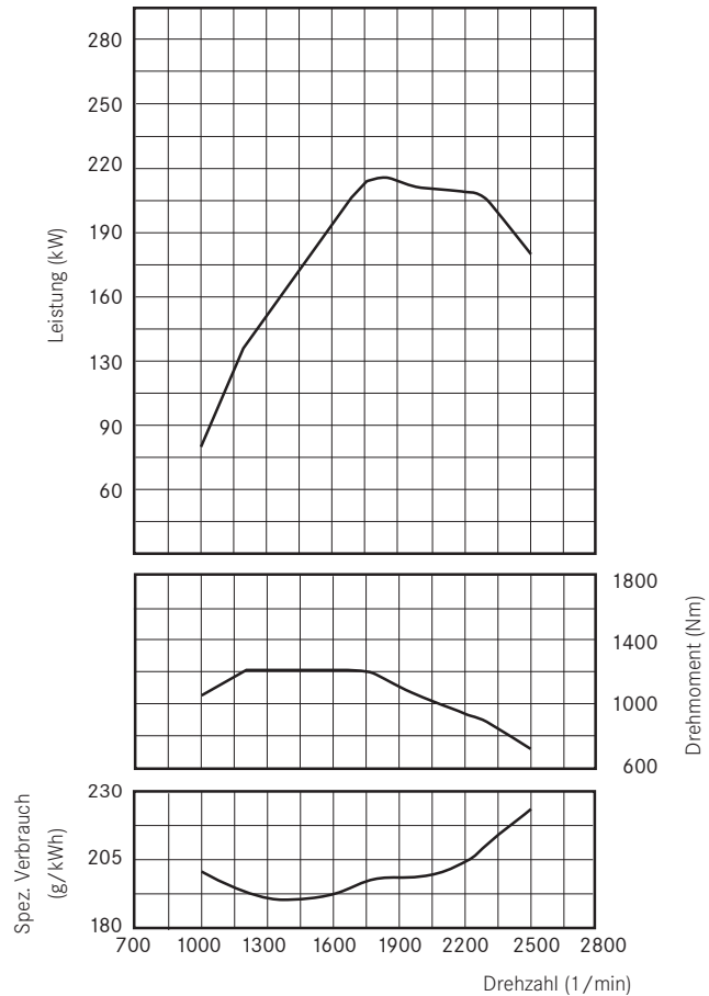
Motor OM 936 h/OM 936 (Euro VI D)
